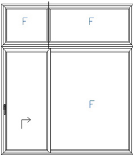
4) 1Vent 3FIX
